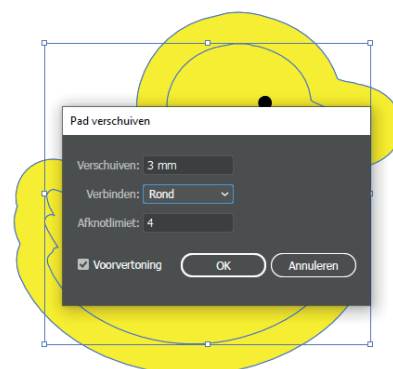
Pad verschuiven
